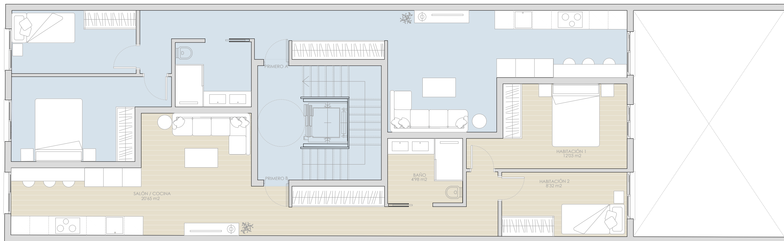
PLANTA PRIMERA
